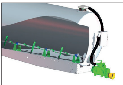
Встроенный миксер с лопастями имеет прямое управление от трактора (в опции).
