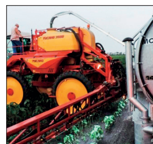
Рукав для заполнения на высоте 4,9 м от земли.
